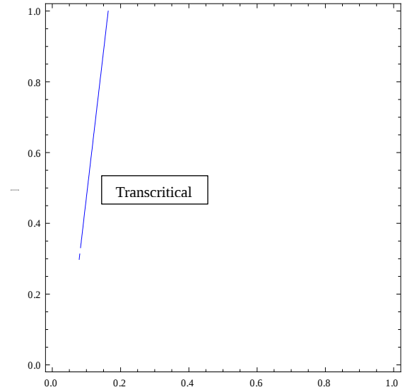
Figure 4: Free Parameters \zeta, \rho
